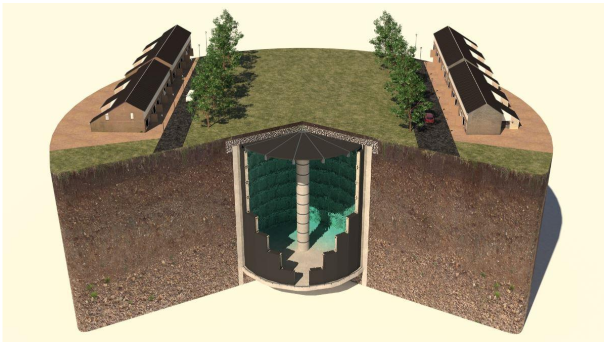
Visual 8.1-1: De Ecovat ondergrondse “thermoskan” in een bestaande woonwijk.
