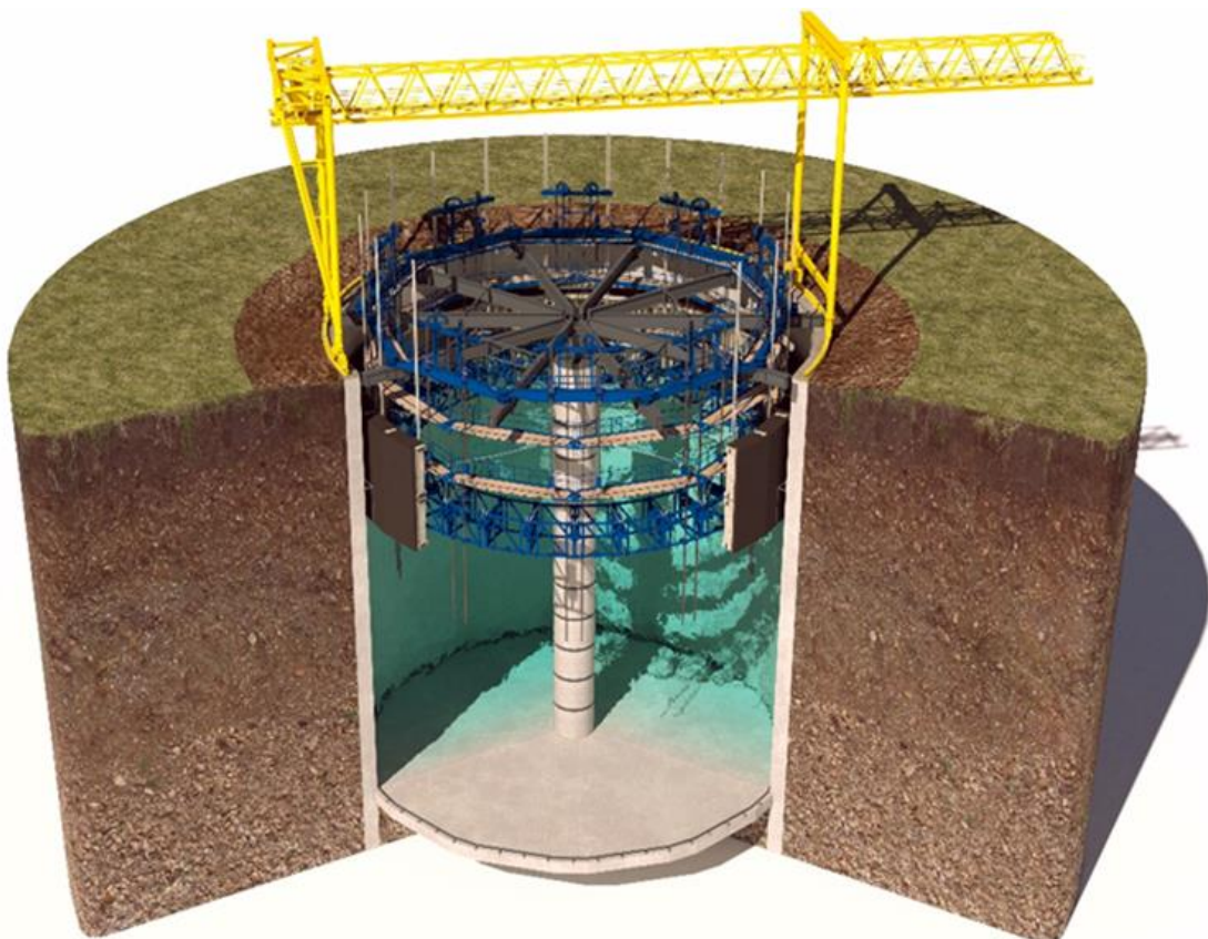
Figuur 9.1-1: Opengewerkt 3D-model tijdens assemblage van het Ecovat. In blauwe kleur het Hijsframe.
